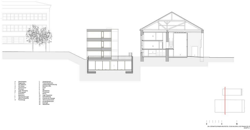
Schnitt DD
