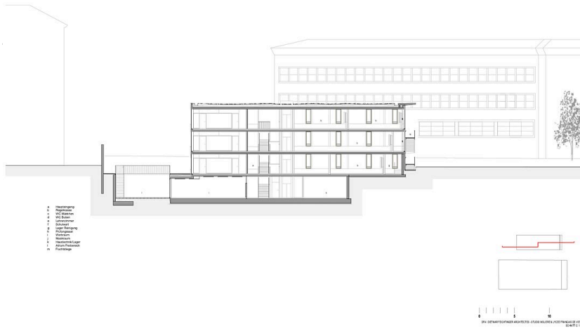
Schnitt CC
