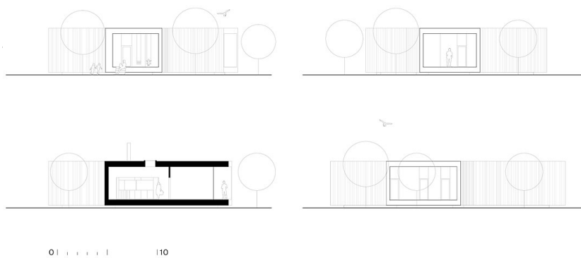
Schnitt und Ansicht
