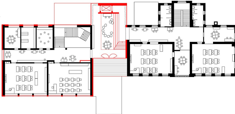
Grundriss OG
