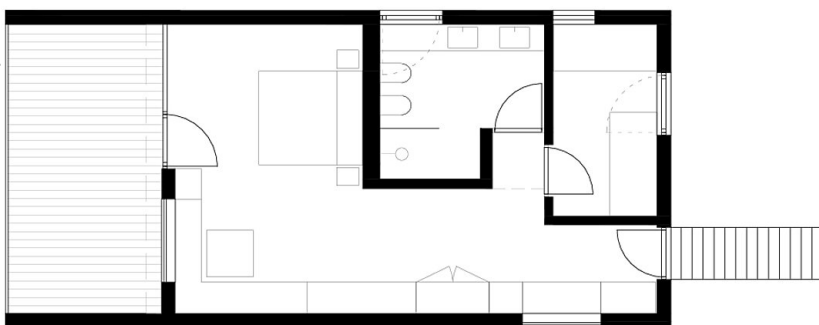
Grundriss Waldhäuser
