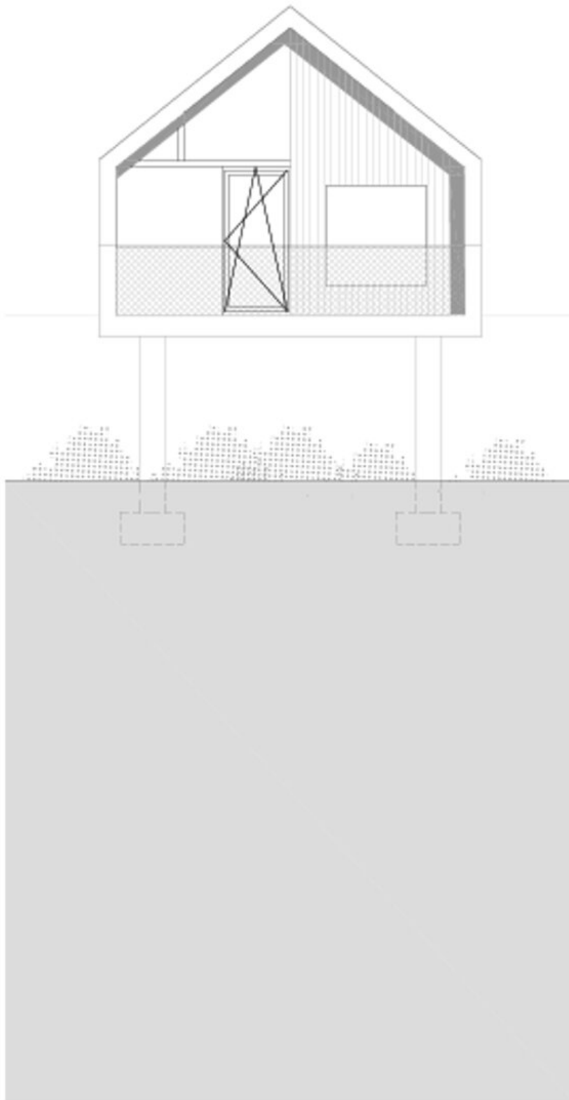
Giebelansicht Waldhäuser
