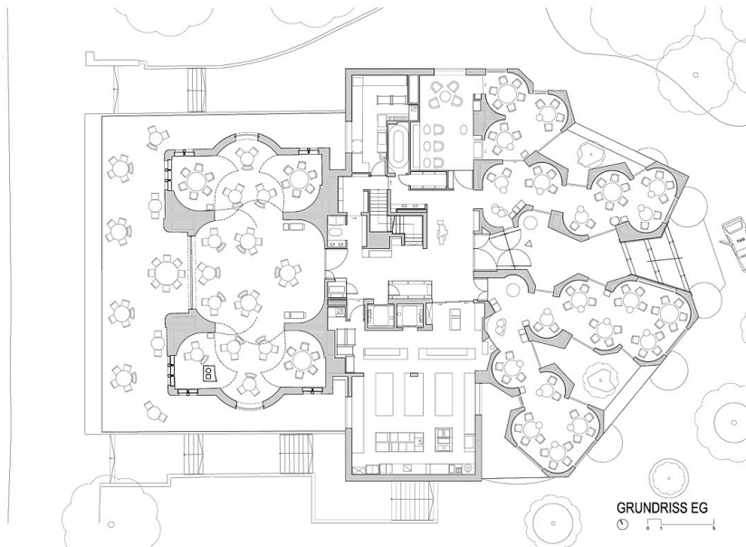
Erdgeschoß
