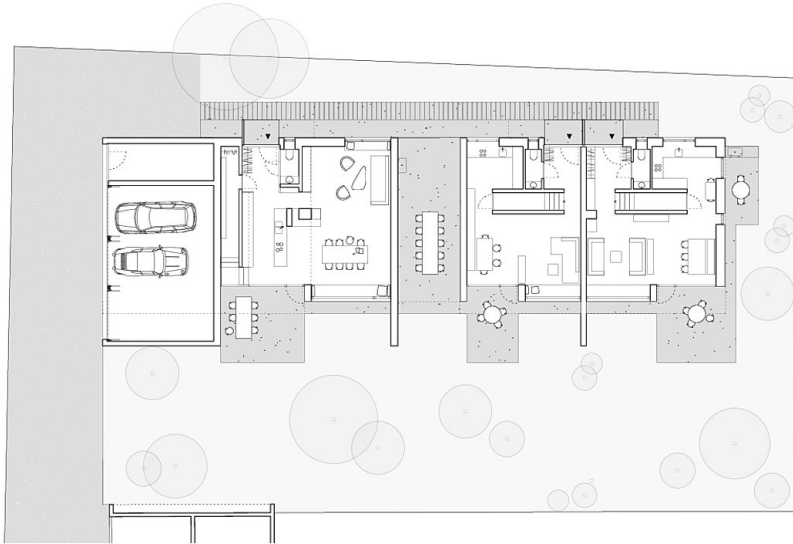
Grundriss EG
