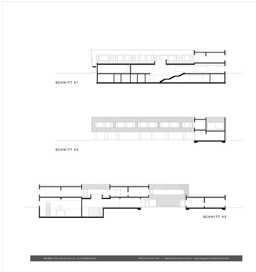
Schnitte
