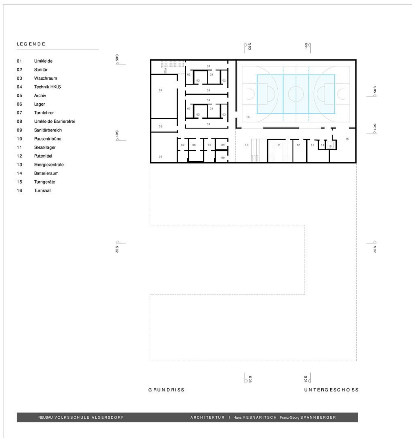
Grundriss UG
