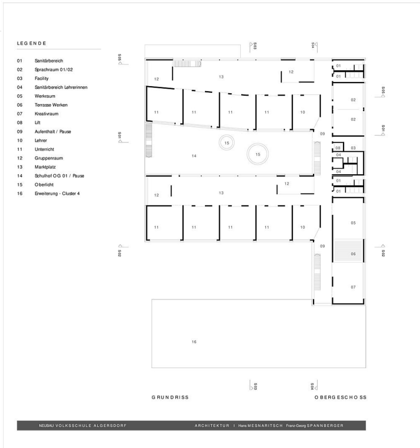
Grundriss OG
