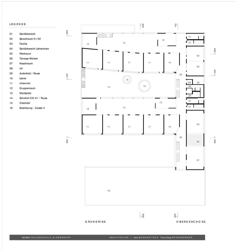
Grundriss OG
