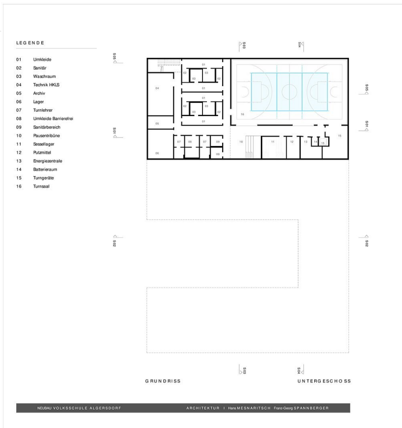
Grundriss UG
