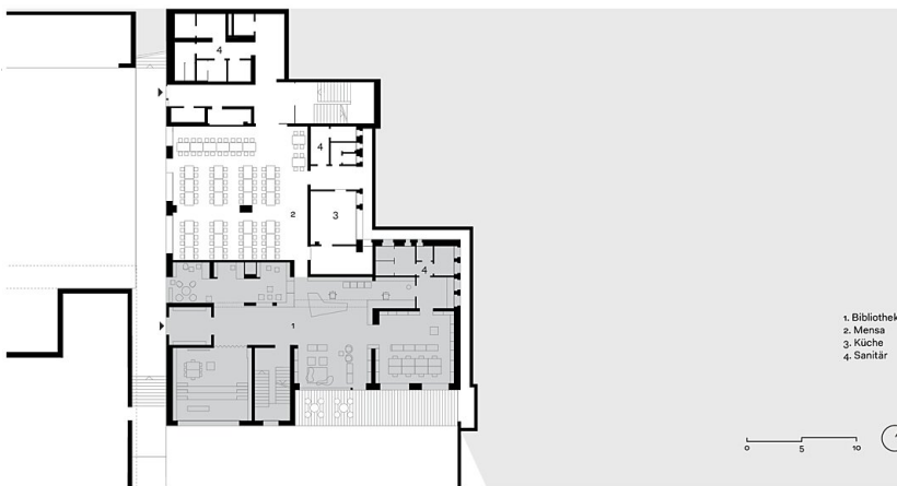
Grundriss UG
