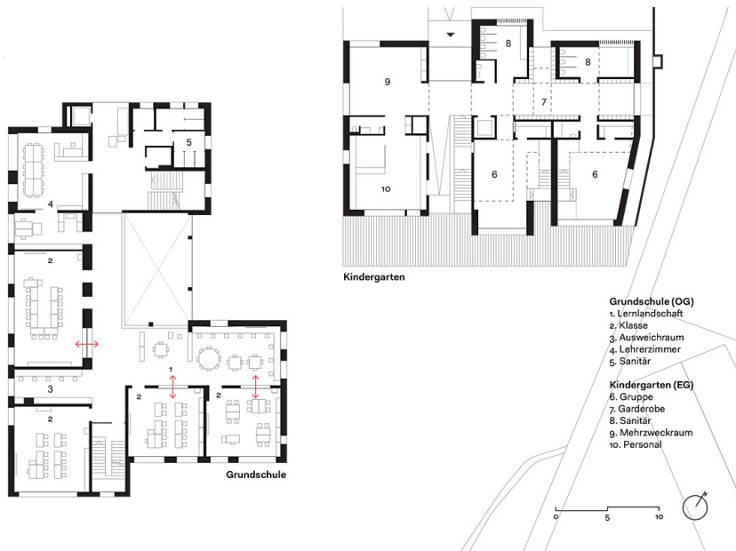
Grundriss OG-EG
