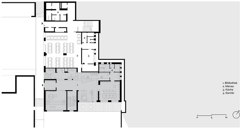
Grundriss UG
