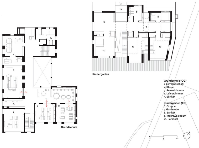
Grundriss OG-EG
