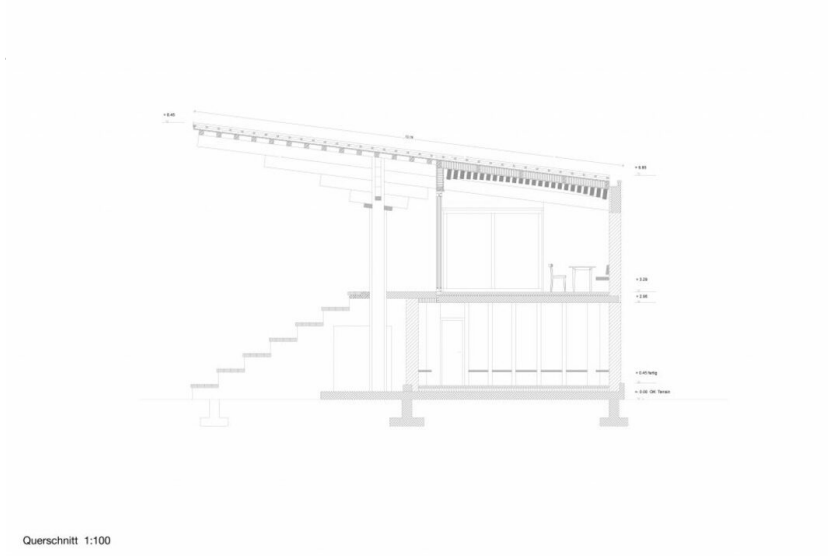
Querschnitt
