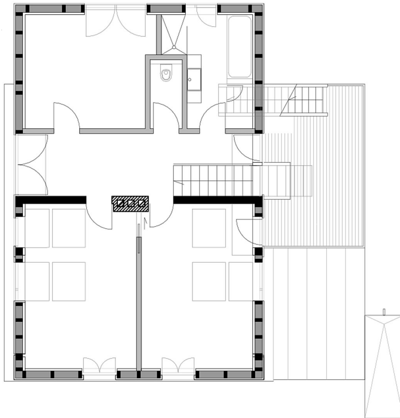
Grundriss DG
