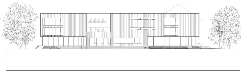
Nordansicht
