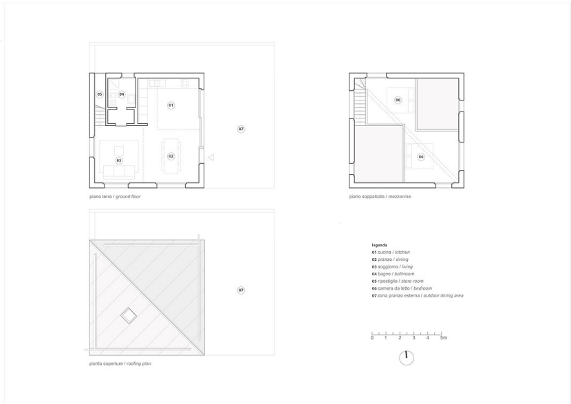
Grundrisse
