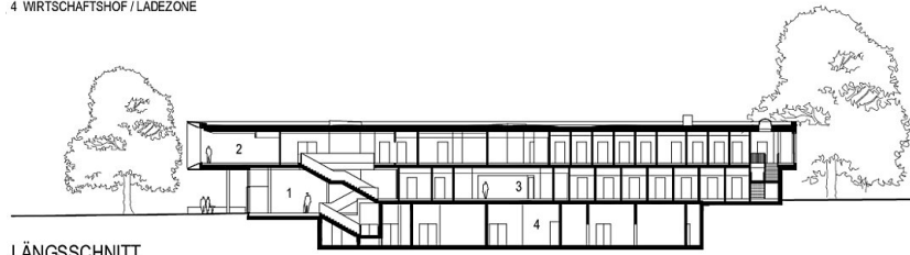
Längsschnitt
