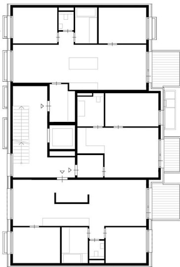
Bauteil D
