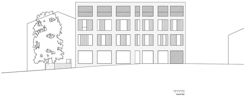
Ansicht Süd
