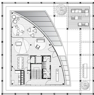
GRUNDRISS OG6 M1:50
