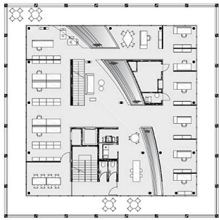
GRUNDRISS OG4
