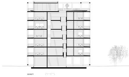
SCHNITT
