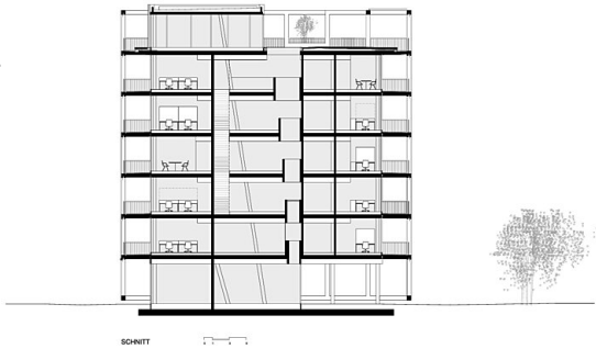
SCHNITT
