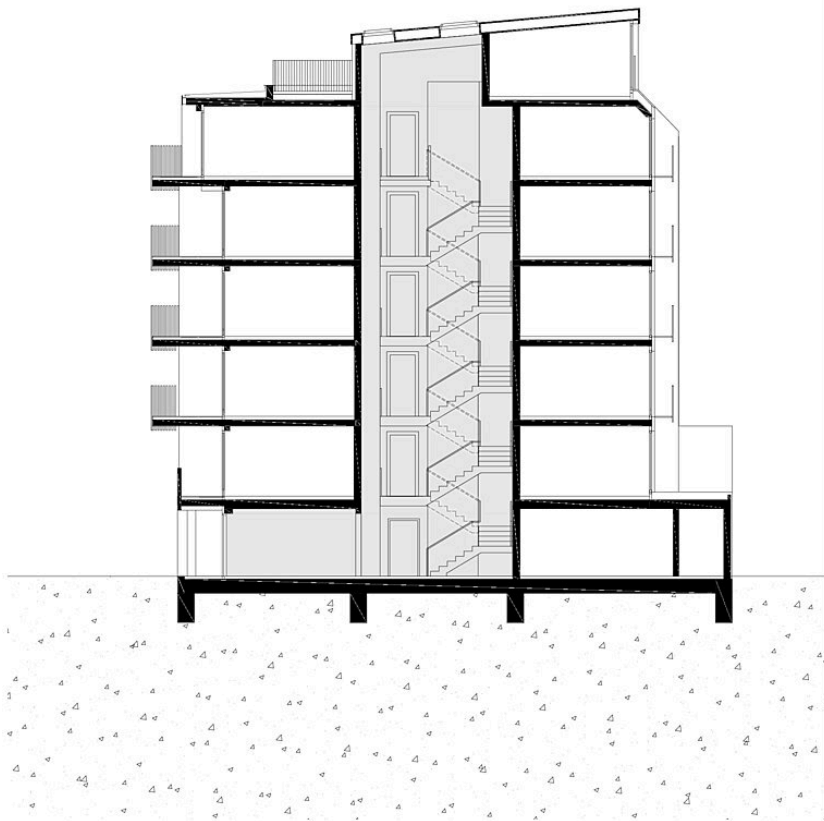
Schnitt
