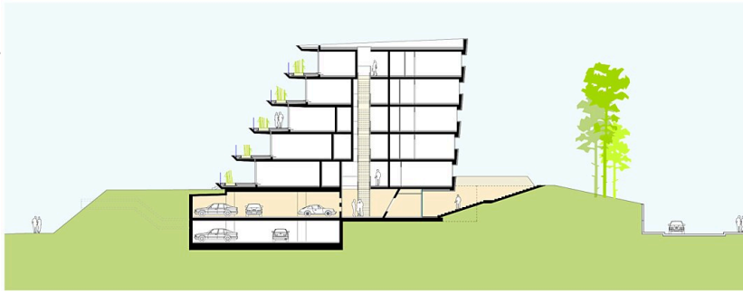
Querschnitt
