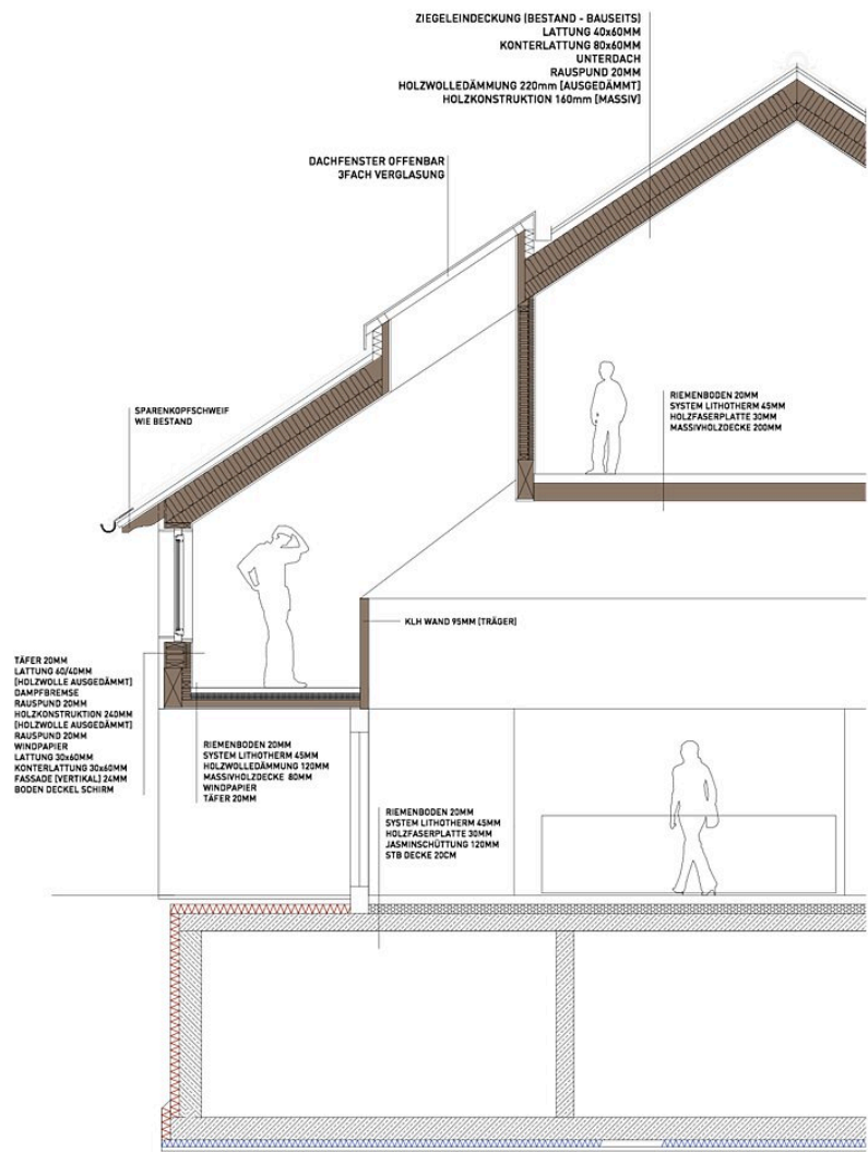
Fassadenschnitt 1: 50
