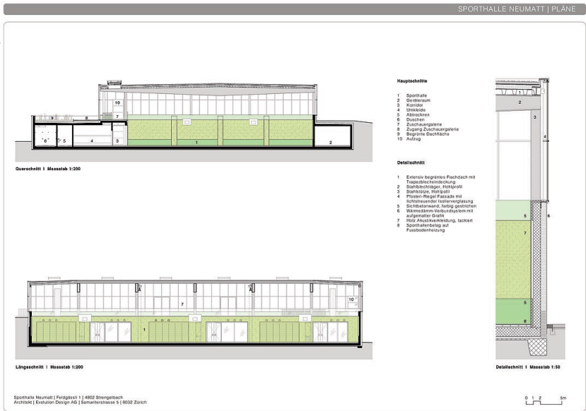
Schnitte
