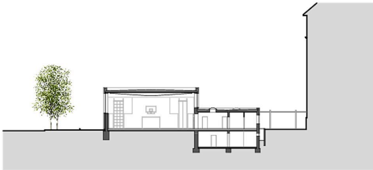
Schnitt
