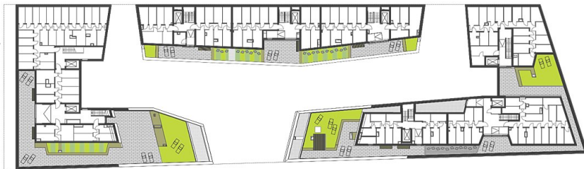
Grundriss Ebene 3
