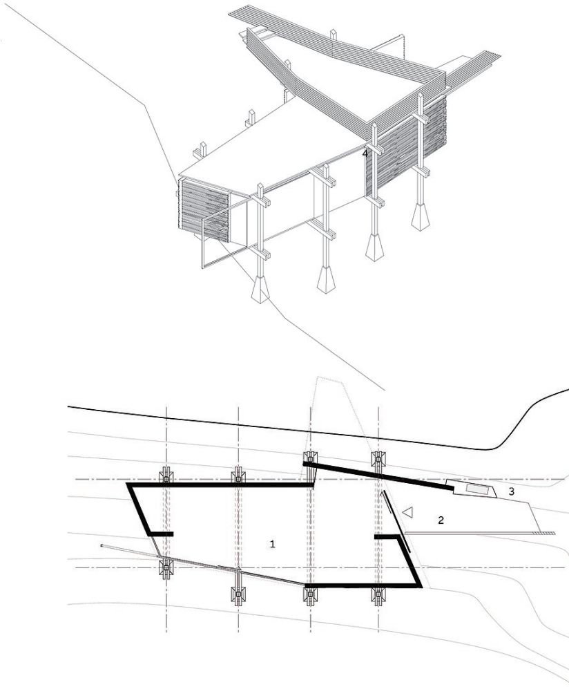
Ansicht, Grundriss
