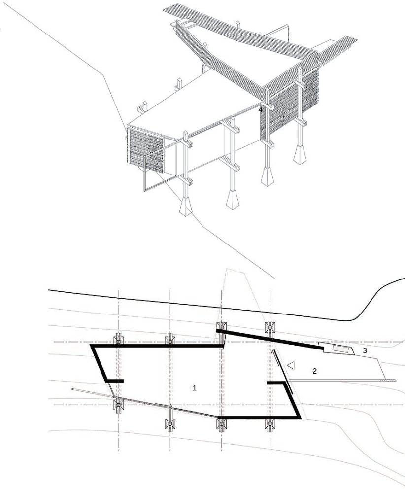
Ansicht, Grundriss
