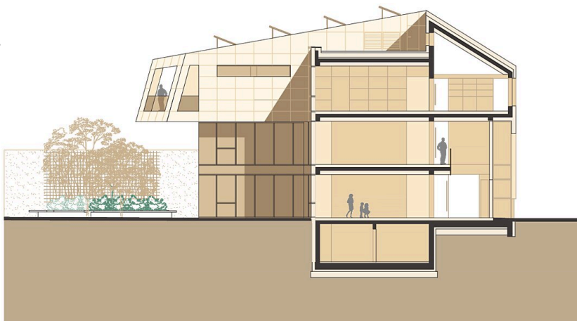
Schnitt Neubau
