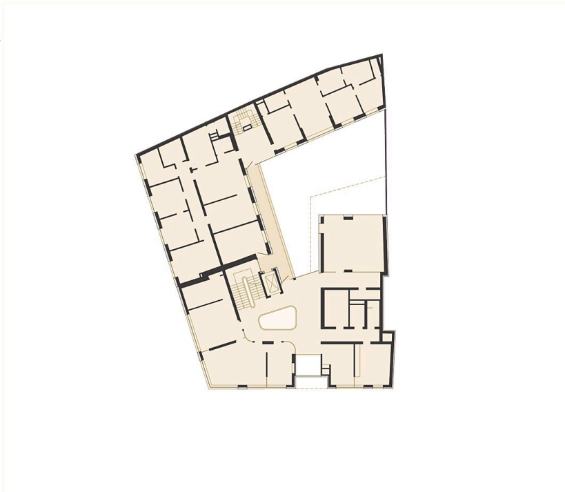
Grundriss OG1
