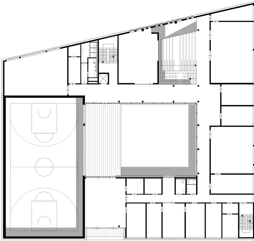
Grundriss OG1
