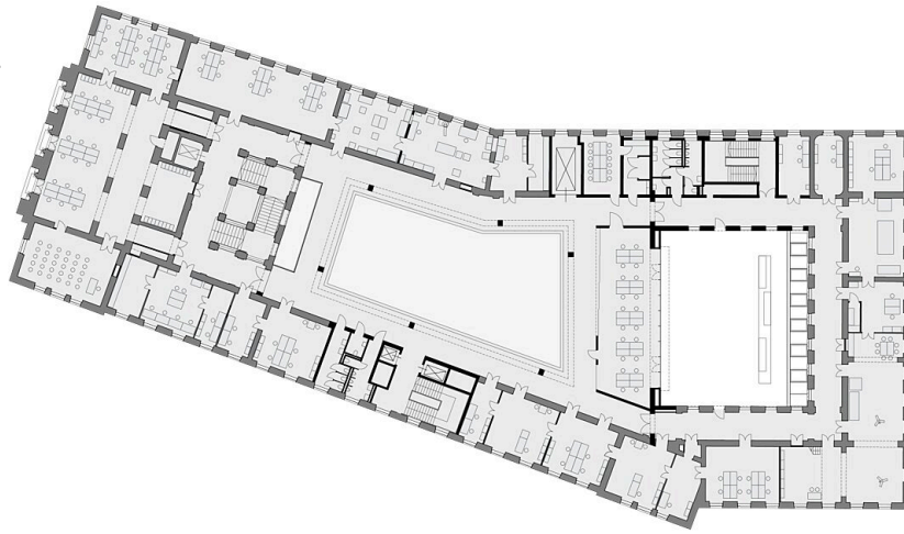
2.Obergeschoss
