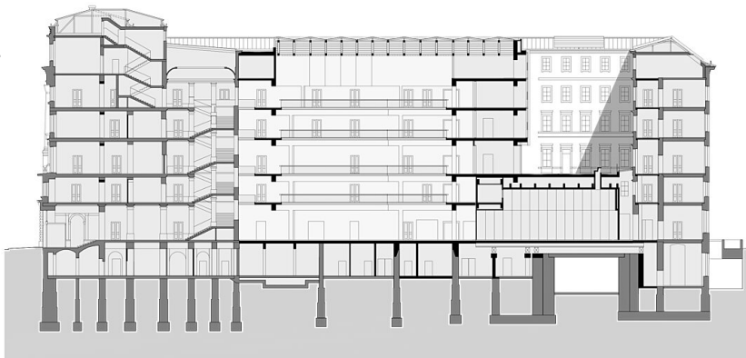
Längsschnitt
