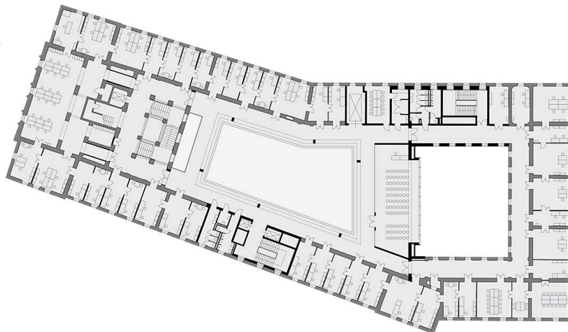
4.Obergeschoss
