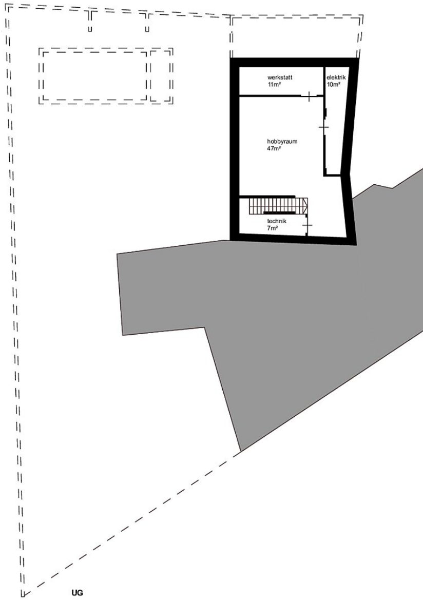
Grundriss UG
