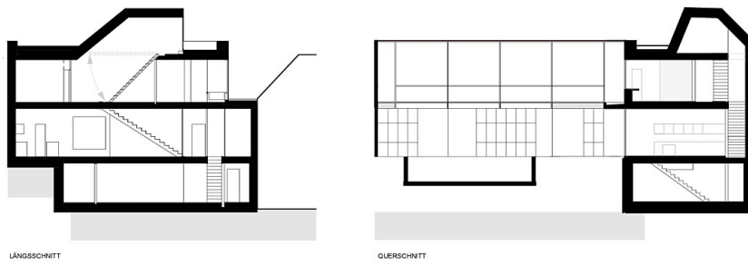
Schnitte
