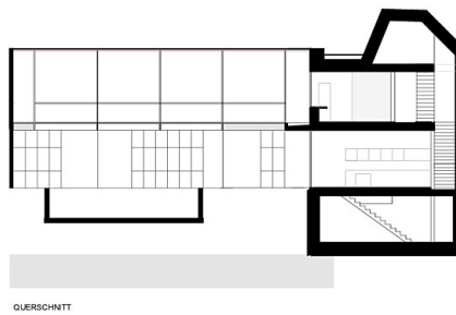
Schnitte
