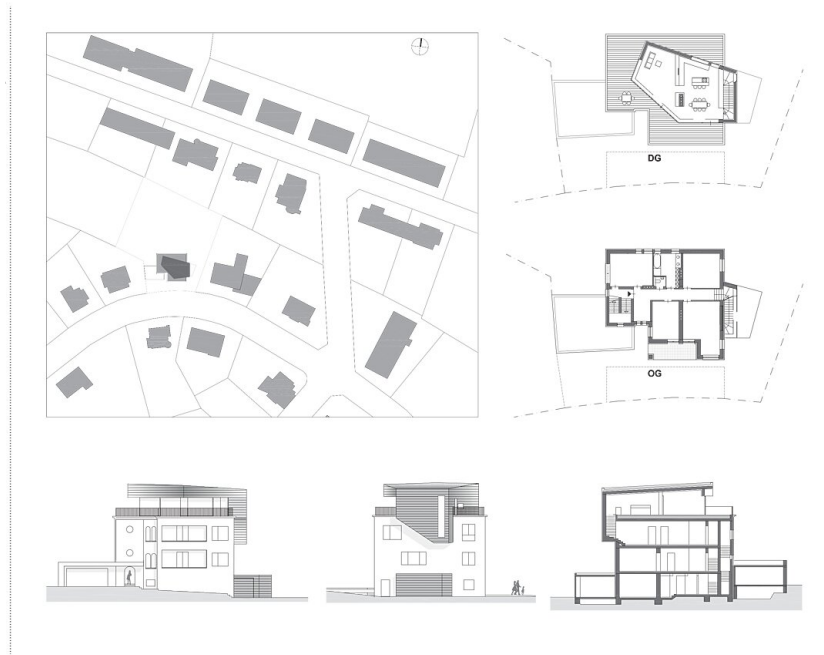
Haus F - Aufbau und Sanierung
