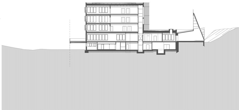
Schnitt 1
