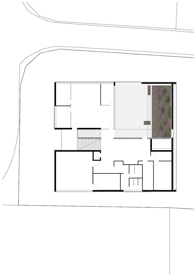
Grundriss OG
