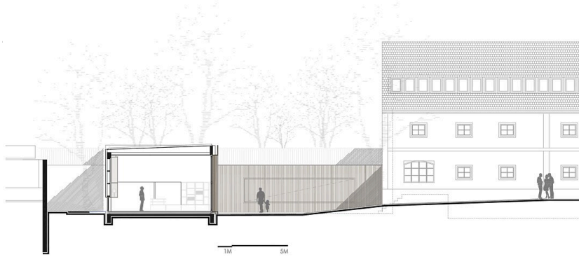
Schnitt B1
