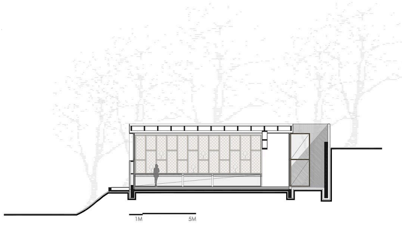
Schnitt A1
