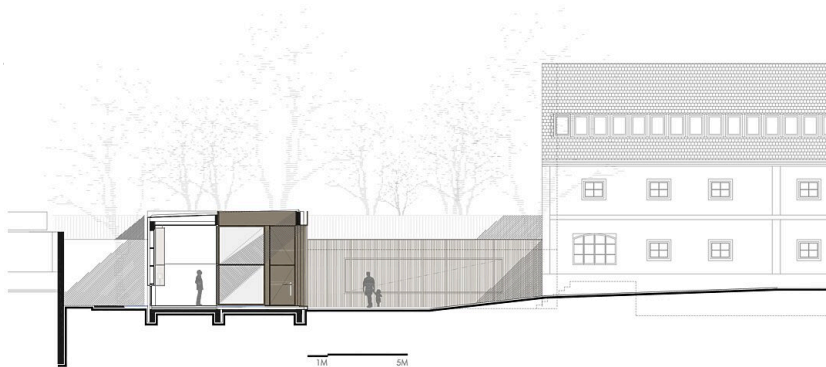
Schnitt B2
