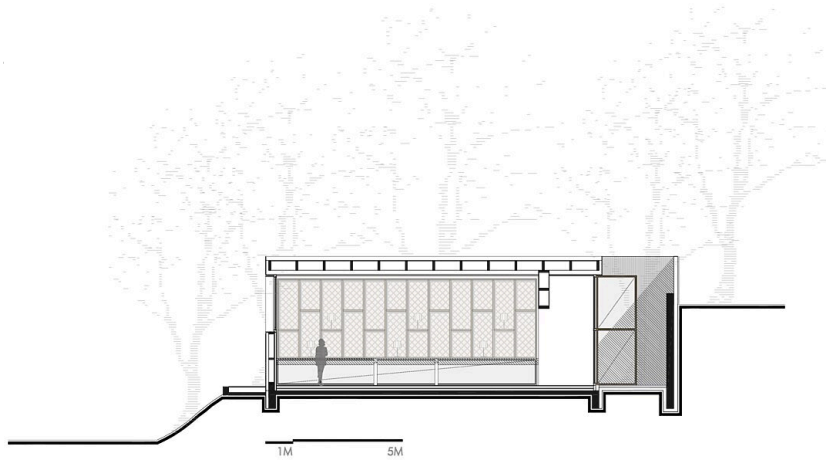
Schnitt A1
