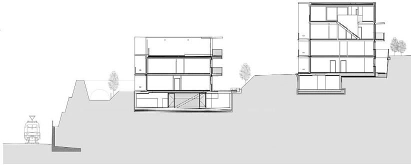
Schnitt 1-1
