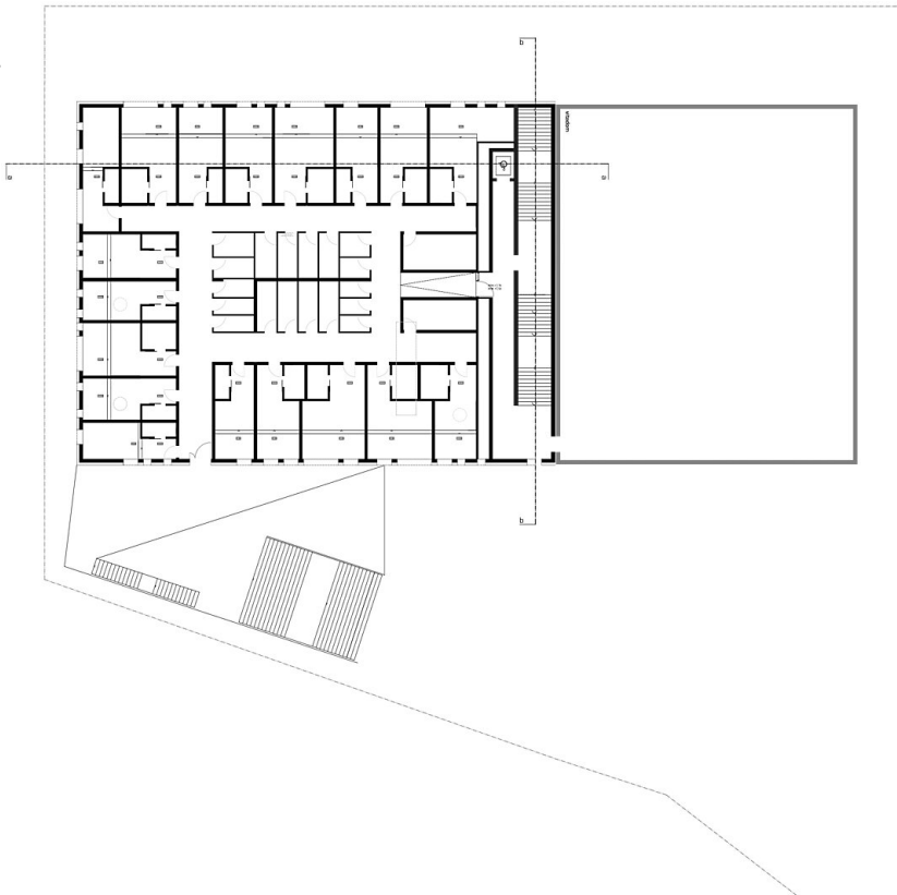
Grundriss OG2
