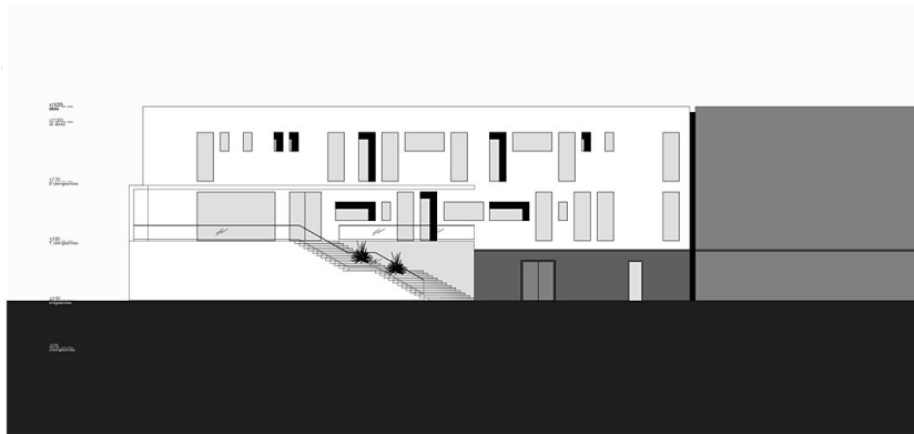
Ansicht Ost
