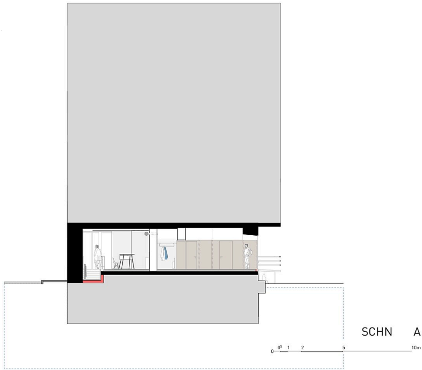
Schnitt A
