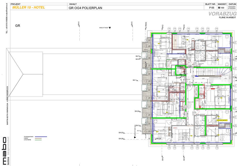
Grundriss OG4
