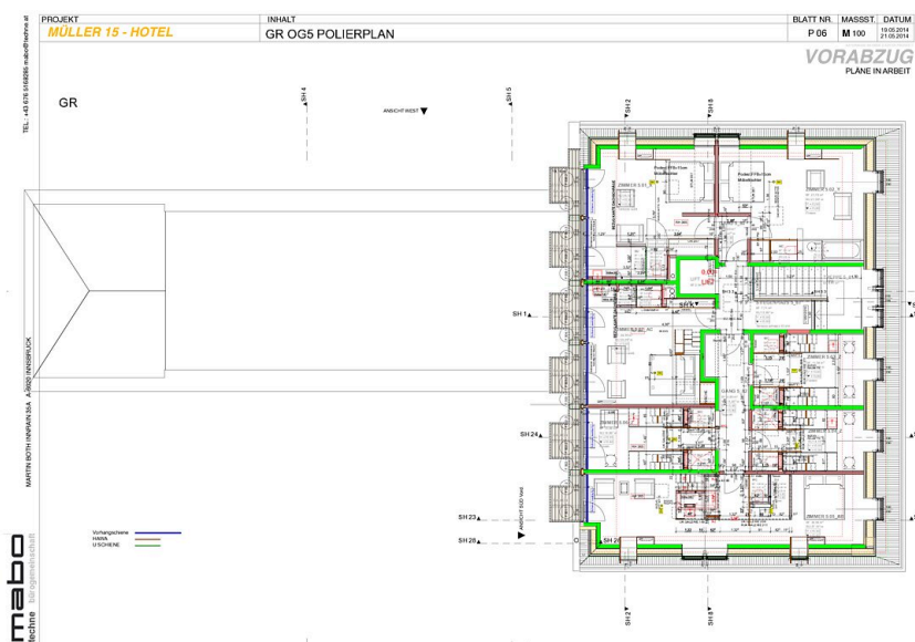
Grundriss OG5
