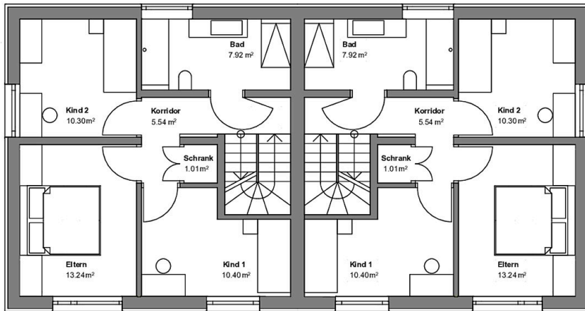
Grundriss OG
