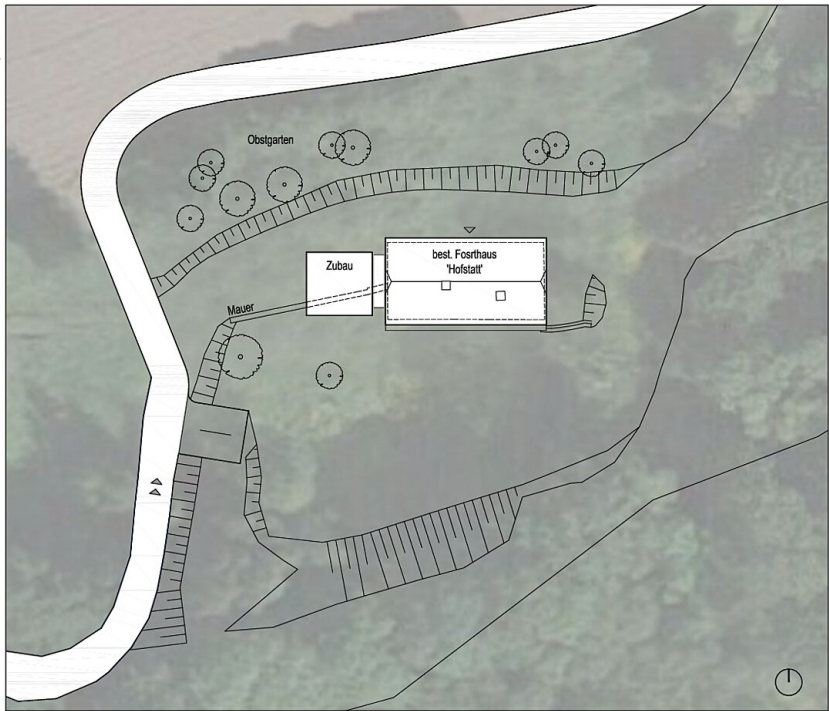
LAGEPLAN 1:500
