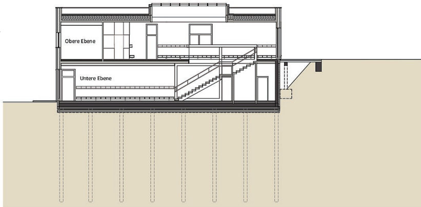
Schnitt M 1:200
