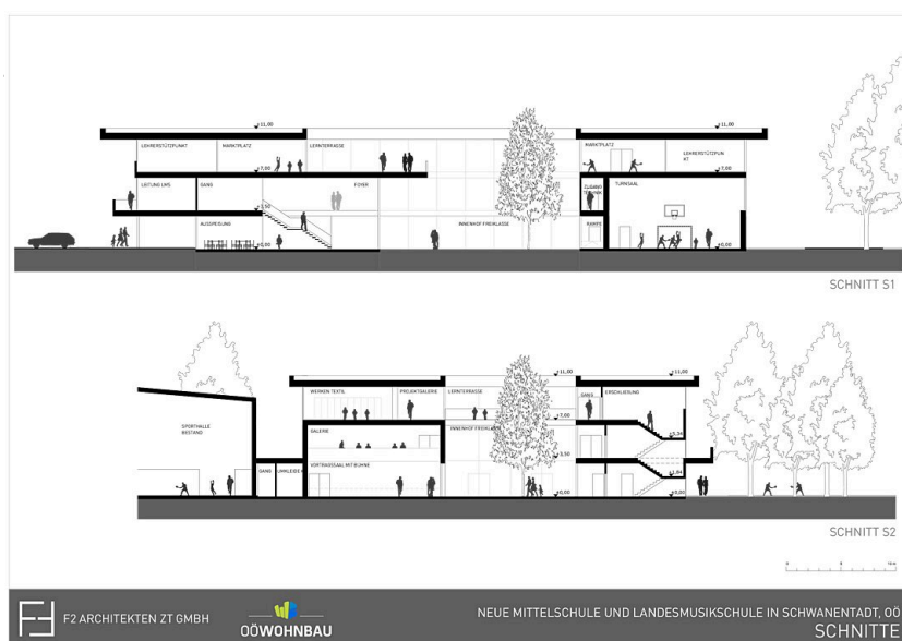
Schnitte
