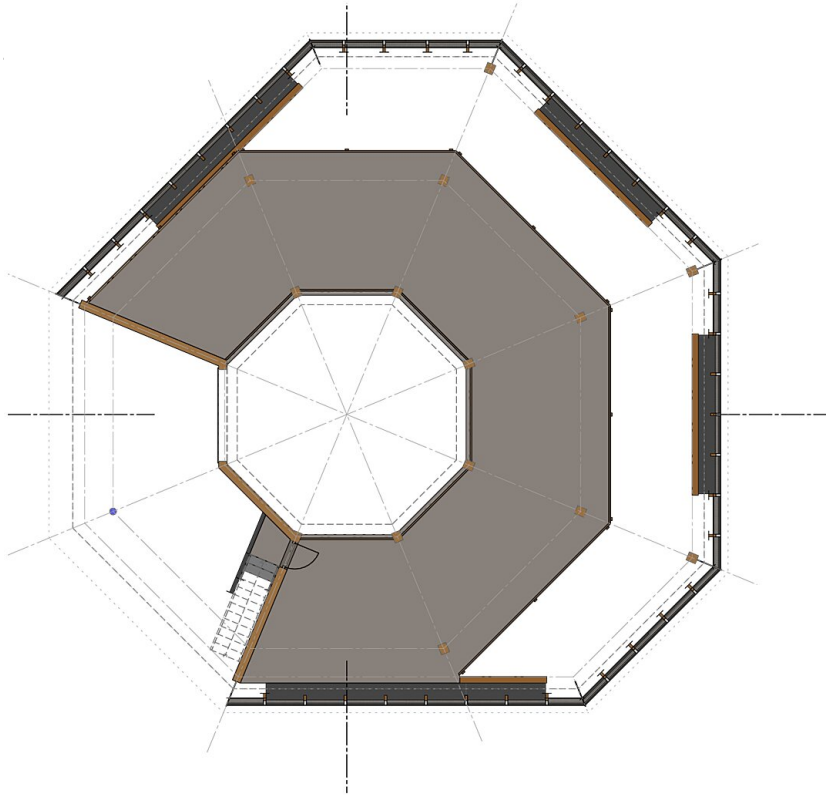
Grundriss OG
