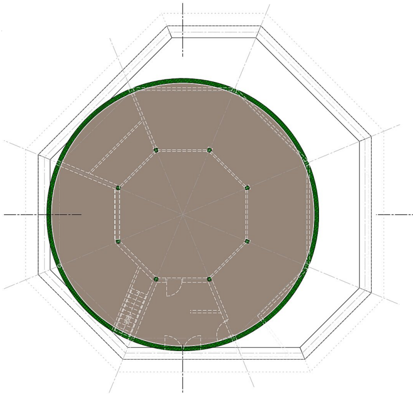
Grundriss UG
