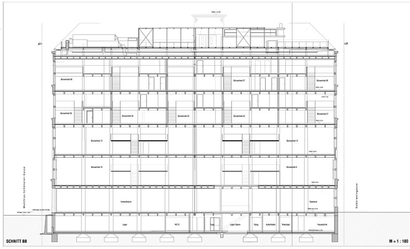
Schnitt B-B
