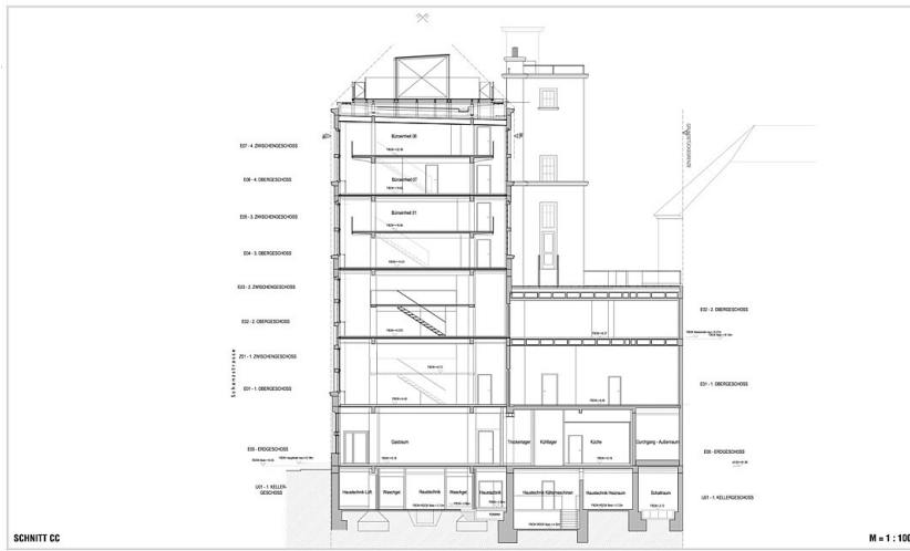
Schnitt C-C
