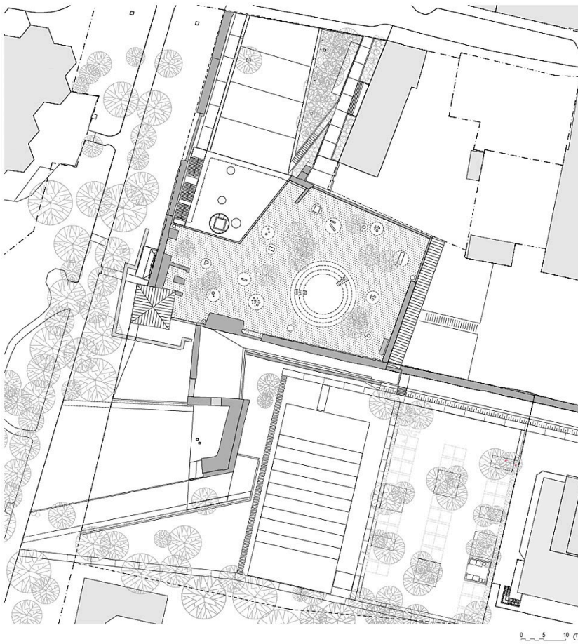
Grundriss DG
