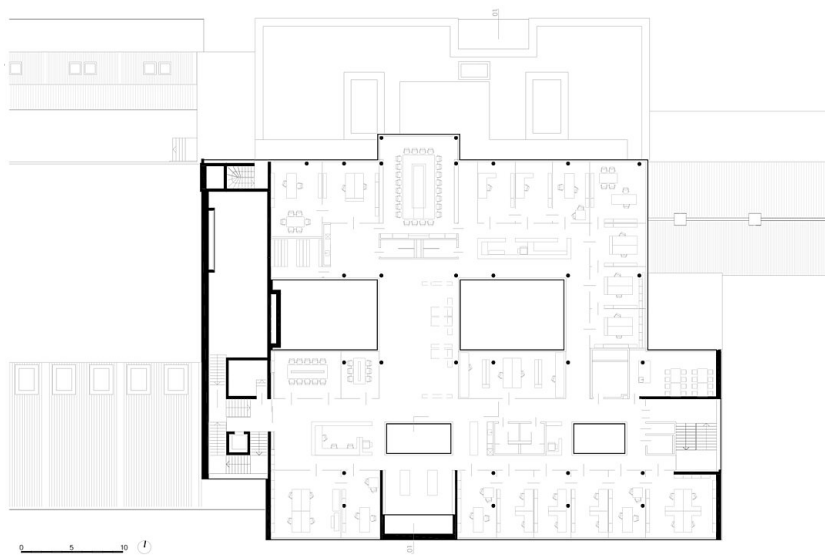
Grundriss
