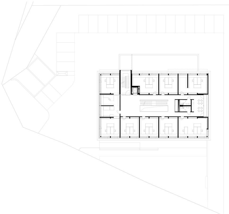
Grundriss OG1
