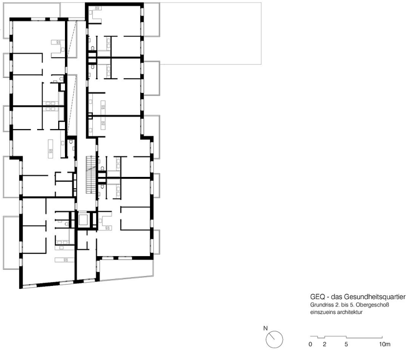
Grundriss RG
