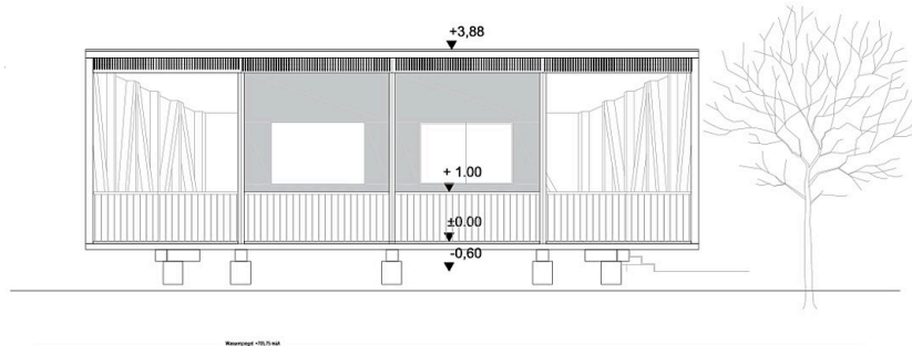
Ansicht Süden 1:100
