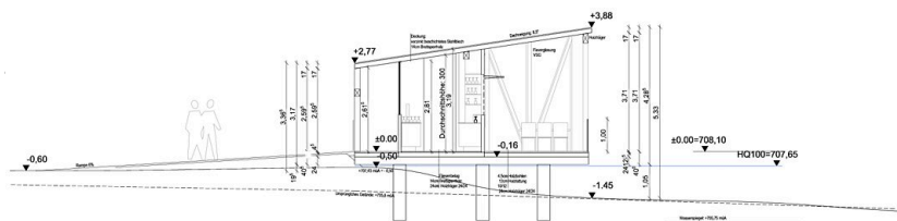
Schnitt B 1:100
