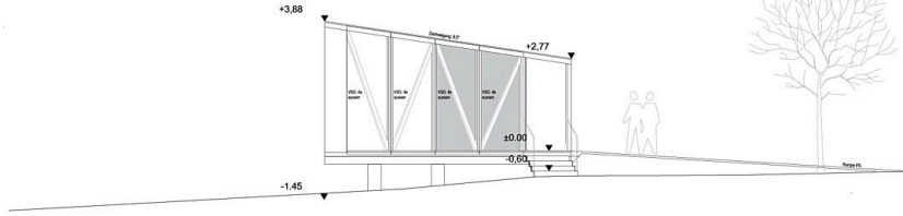
Ansicht Osten 1:100
