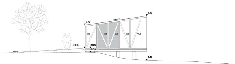
Ansicht Westen 1:100
