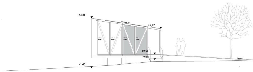
Ansicht Osten 1:100
