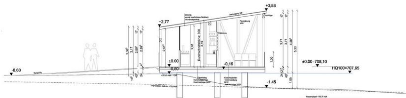
Schnitt B 1:100
