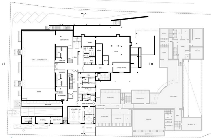
ZV-Bauherrpreis Grundriss Untergeschoss | 1:200 thalmeier architektur ZT GmbH Fuchsbweg 12 | 4430 Bad Ischl | www.thalmeier.at 5400 Haiden | Tel. +43(0)62 43182 340 | office@thalmeier.at 5400 Haiden | Fax +43(0)62 43182 300-40
