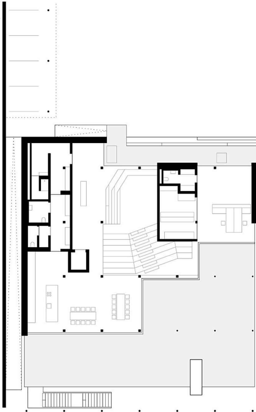
Grundriss OG
