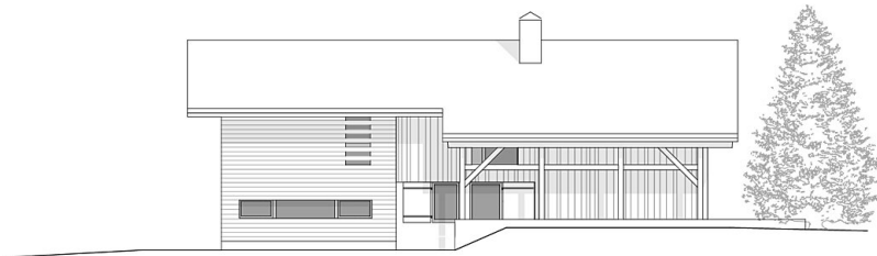
Ansicht Nordwest 1:100
