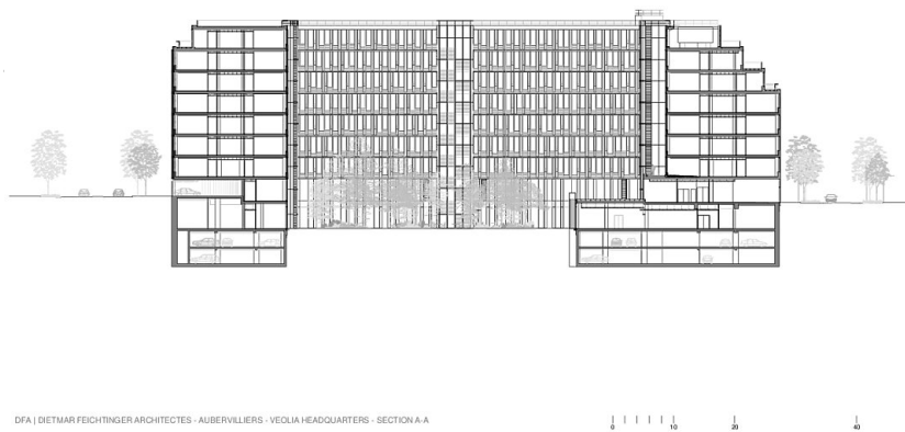
Schnitt AA
